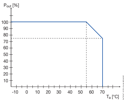
CP-D 24/2.5
