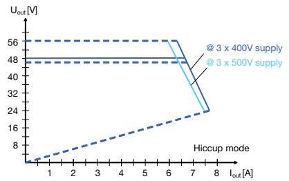
CP-T 48/5.0
