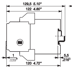
CC-U/x , CC-U/xR
