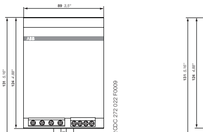
CP-T 24/10.0, CP-T 48/5.0
